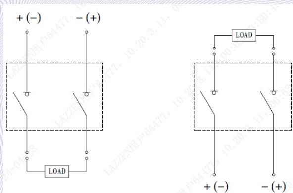
2P 外形接线图(DC1500V):
